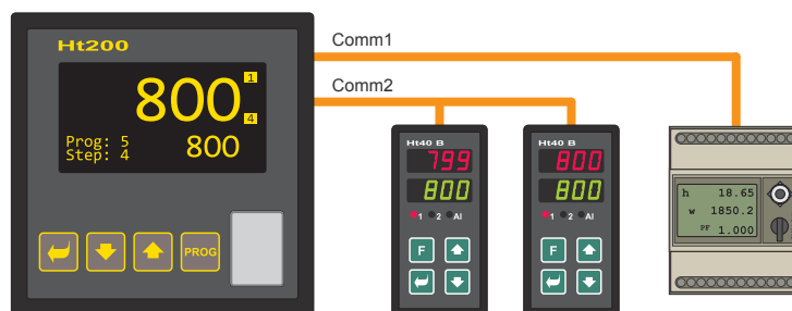
Příklad záznamu dat v dataloggeru u systému „Master - Slave“ se 2 podřízenými regulátory a měřičem energie
