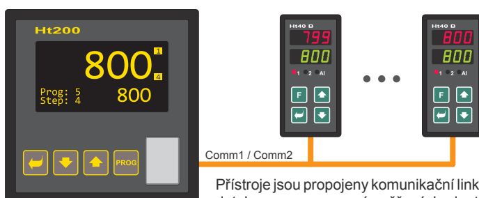
Příklad záznamu dat v dataloggeru u systému „Master - Slave“ se 7-mi podřízenými regulátory
